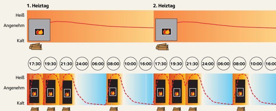
RAUMTEMPERATUREN BEI VERSCHIEDENEN OFENTYPEN.
